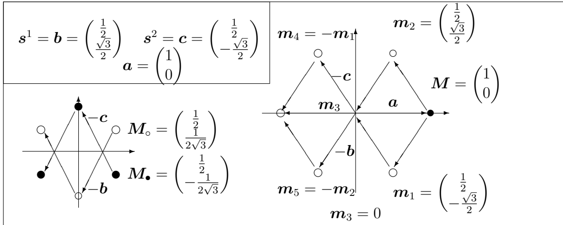
Slika 4.5: \mathfrak{sl}(3, \mathbb{C}) : fundamentalne ( M_{\circ} = \begin{pmatrix} \frac{1}{2} \\ \frac{1}{2\sqrt{3}} \end{pmatrix} i M_{\bullet} = \begin{pmatrix} \frac{1}{2} \\ -\frac{1}{2\sqrt{3}} \end{pmatrix} ) i pridružena reprezentacija.
