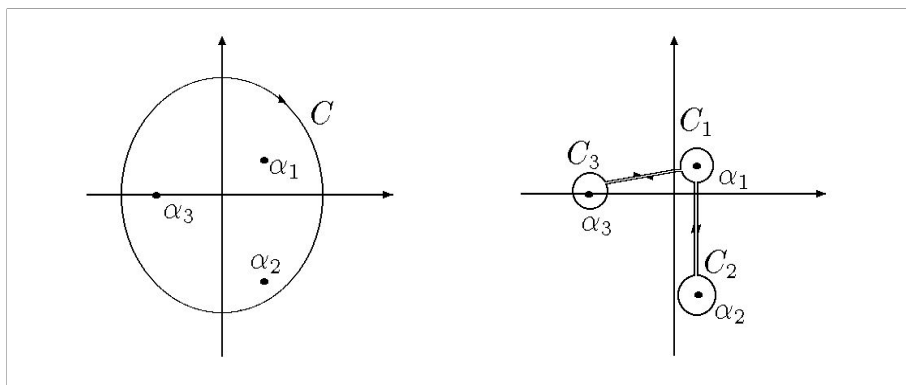
Slika 2.3: Sažimanje konture integracije oko svojstvenih vrednosti.
