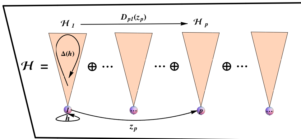
Slika 3.5: Geometrija indukcije. Osnovno dejstvo (osnova slike) na nekoj orbiti sa stabilizatorom H (elementi h ), odnosno grupno množenje kad se tačke orbite identifikuje sa transverzalom (elementi z_p ), "podigne" se u vektorski prostor \mathcal{H} koji je raslojava u direktni zbir potprostora (slojeva) nad tačkama orbite.
