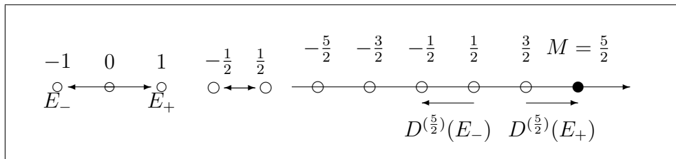
Slika 4.4: sl(2, \mathbb{C}) : korenovi i težine pridružene (ireducibilna sa M = 1 ), fundamentalne ( M = \frac{1}{2} ) i reprezentacije M = \frac{5}{2} .
